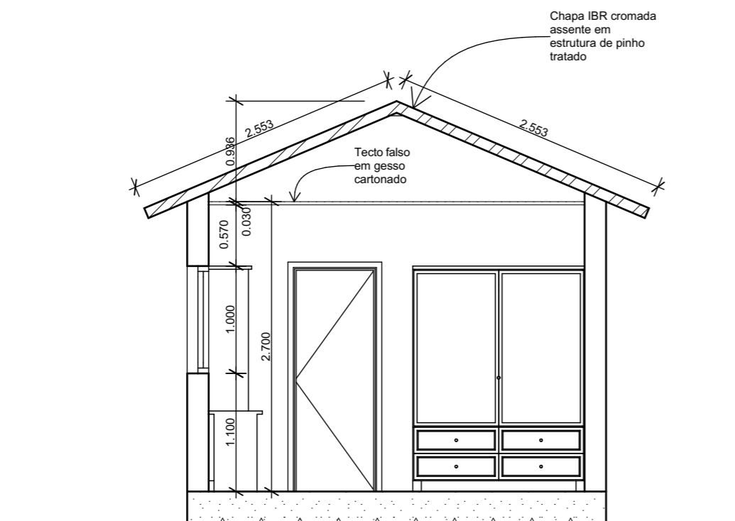
CORTE S-01 esc.:1/50
