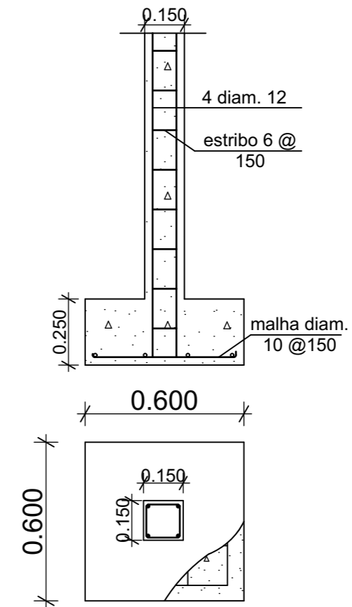
PORMENOR SAPATA/PILAR esc.:1/20
