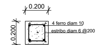
VIGA DE FUNDAÇÃO NÍVEL DO PAVIMENTO esc:1/20
