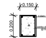
VIGA DE COROAMENTO COTA 2,10 esc:1/20
