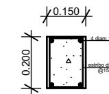
Viga de coroamento
