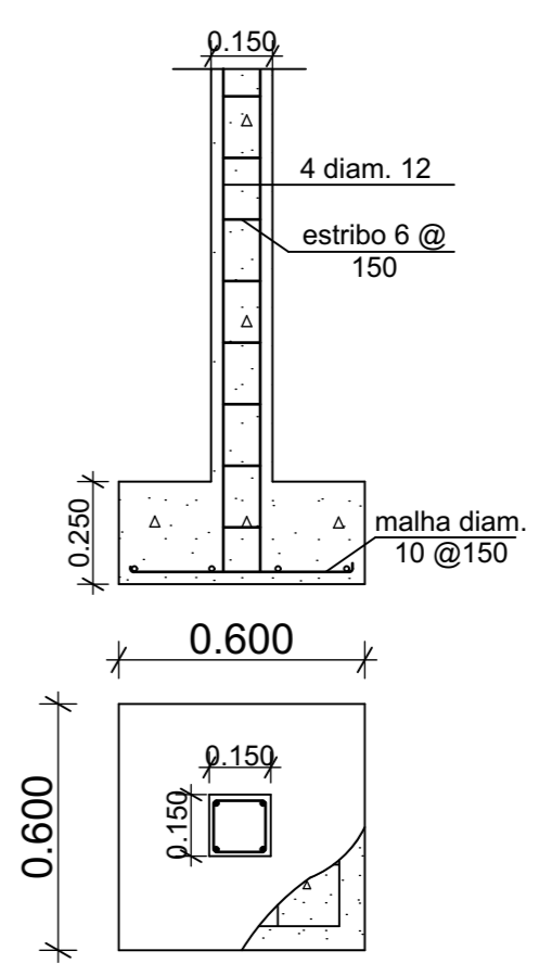
Detalhe sapata/pilar
