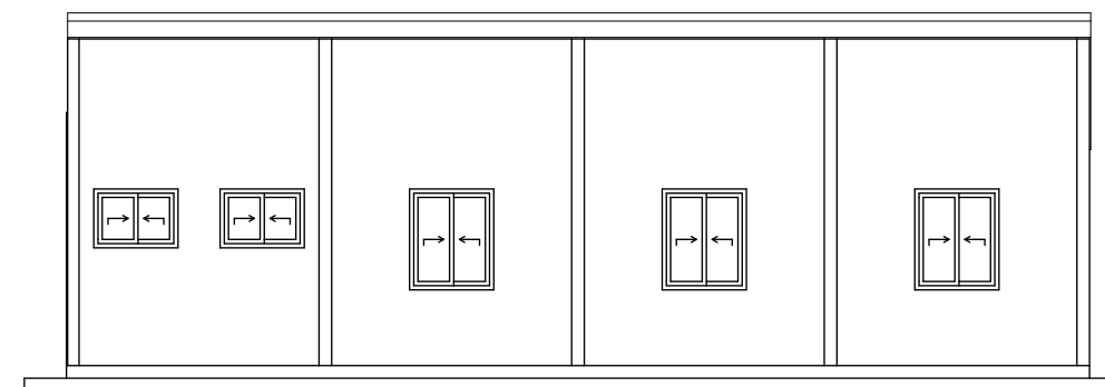
ALÇADO POSTERIOR
