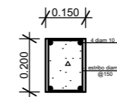
VIGA DE COROAMENTO COTA 2,10 esc:1/20
